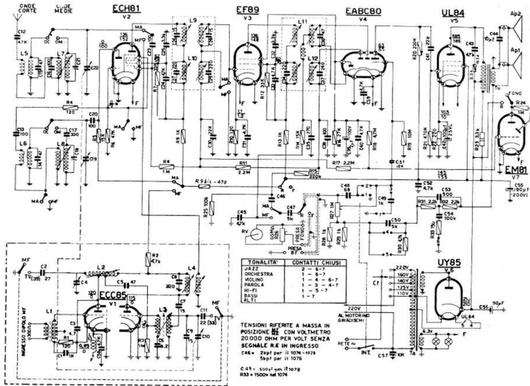
RADIORICEVITORI ALLOCCHIO BACCHINI Modd. 1074 - 1076 - 1078
